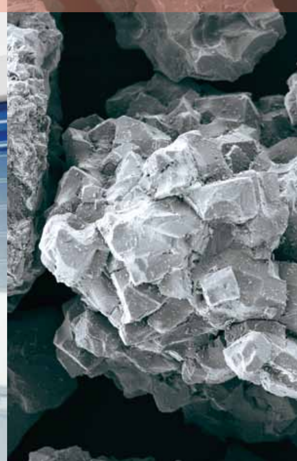
REM-Analyse.
